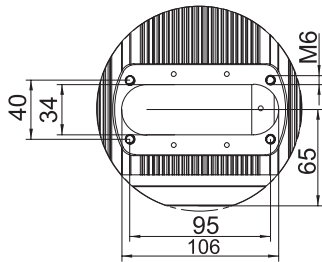
Ansicht Z / View Z
